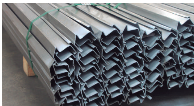
MARCO PUERTA TIPO ALUMINIO Espesores: 085 mm, 1,00 mm y 1,10 mm
